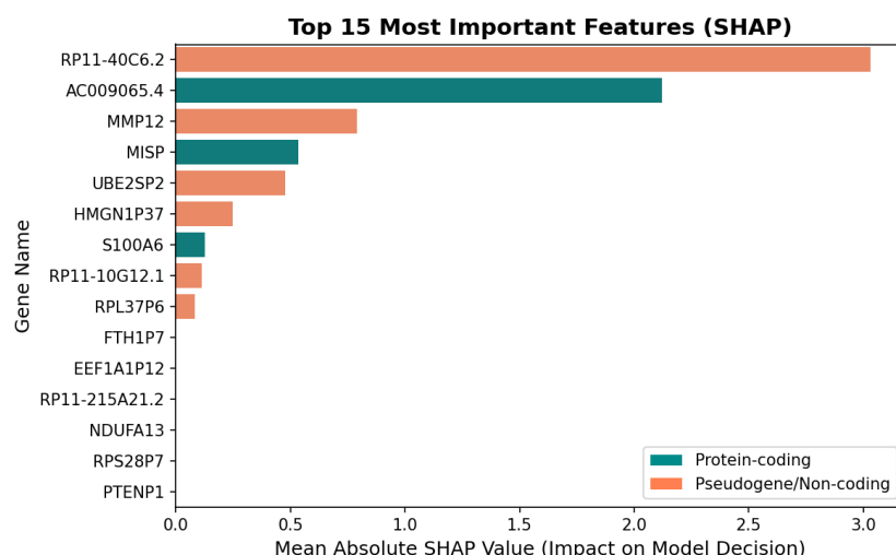
Figure 2: SHAP 摘要圖，顯示推動 L1 邏輯斯迴歸分類器決策的前 15 個特徵重要性排名。
